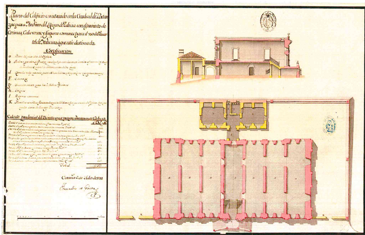
Plano del Edificio construido en la Ciudad de Betanzos para Archivo del Reino de Galicia con el proyecto de Cocinas, Calavozos, y lugares comunes para el uso del Cuartel de milicias, á que esta destinado
